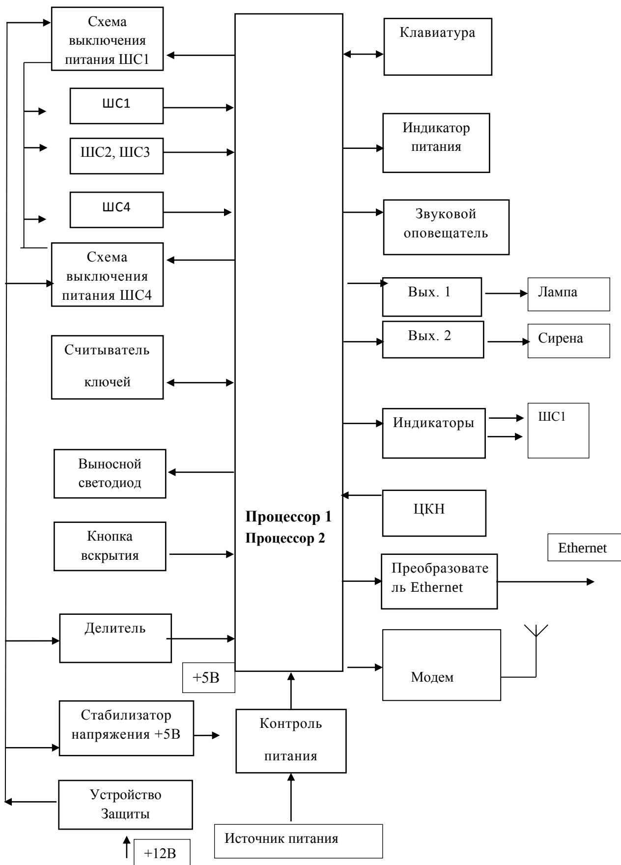
Структурная схема прибора «Лагуна-IP/GSM»
